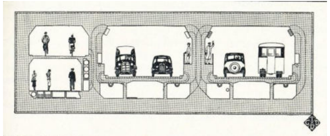
Een schets van de dwarsdoorsnede van de Maastunnel.
