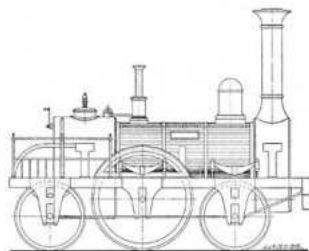
DE HOOP, evenals DE SNELHEID gebouwd door Longridge en Cie te Bedlington.
